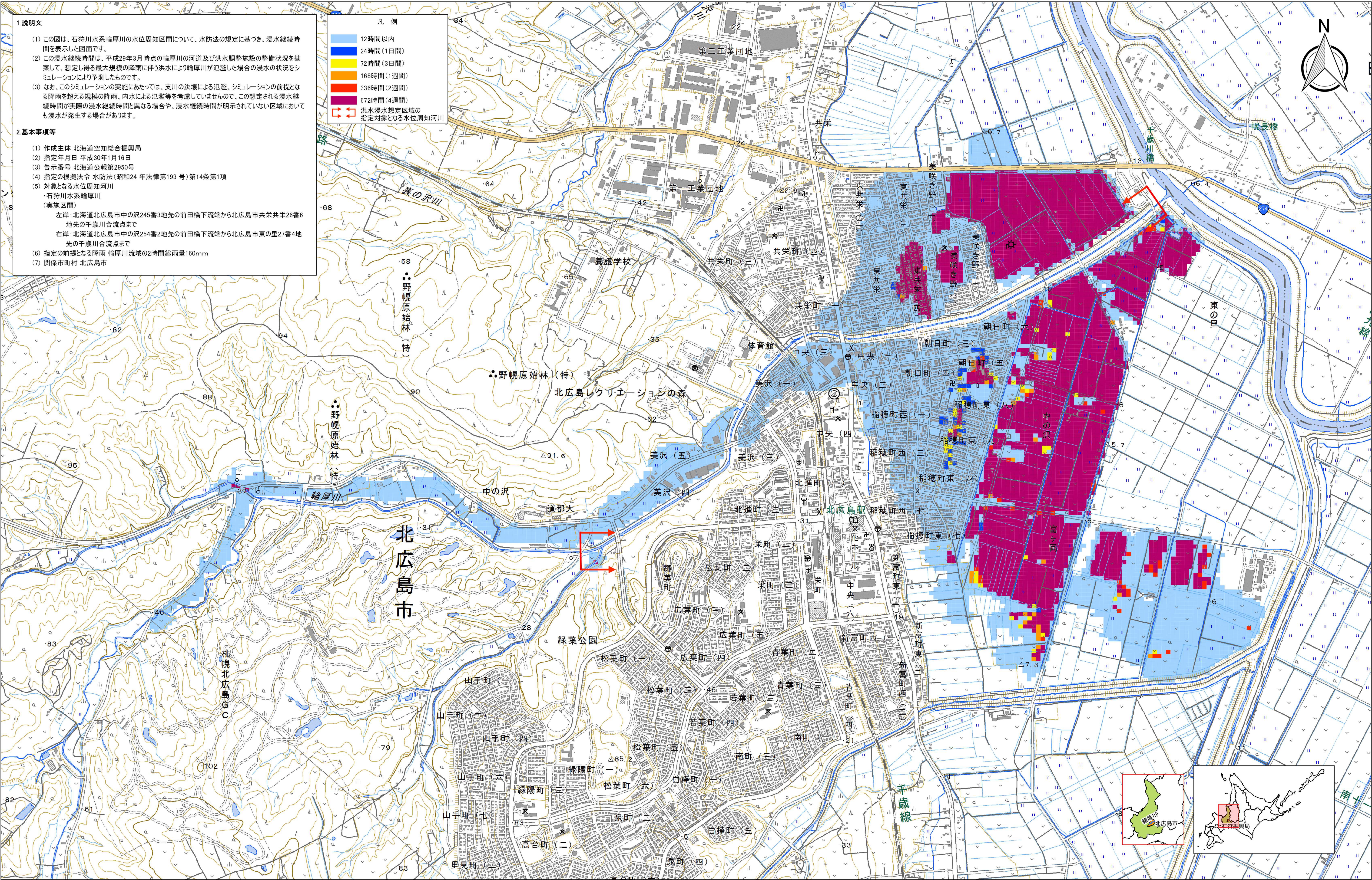
石狩川水系輪厚川 浸水継続時間(想定最大規模)
