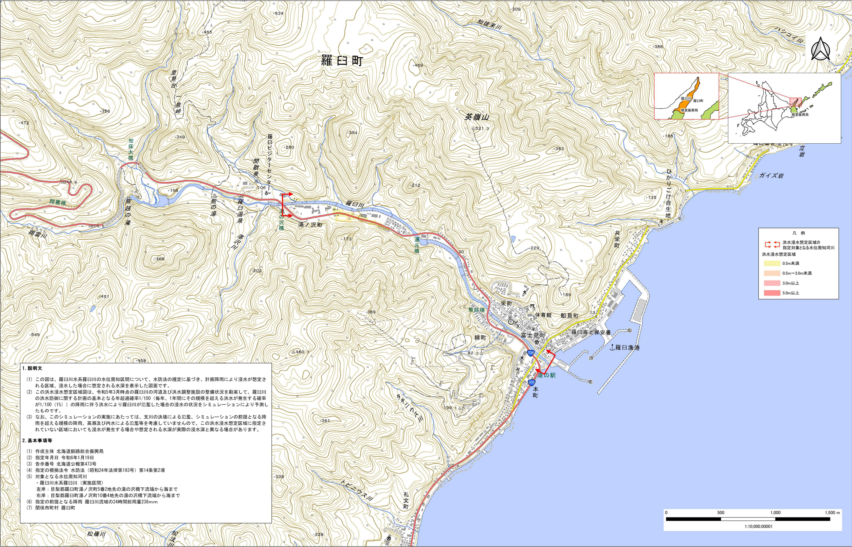
羅臼川水系羅臼川 洪水浸水想定区域（計画規模）
