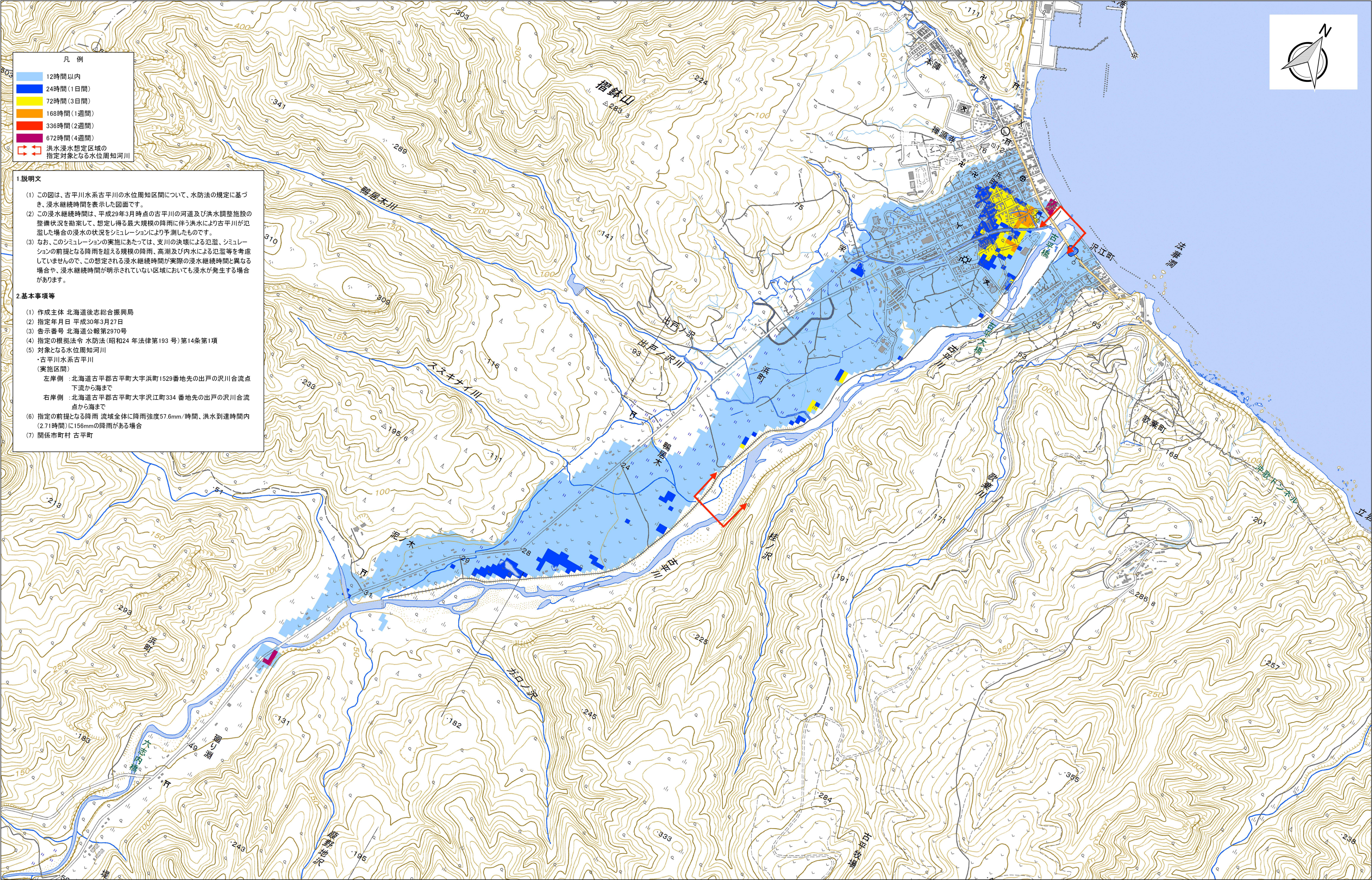
古平川水系古平川 浸水継続時間(想定最大規模)
