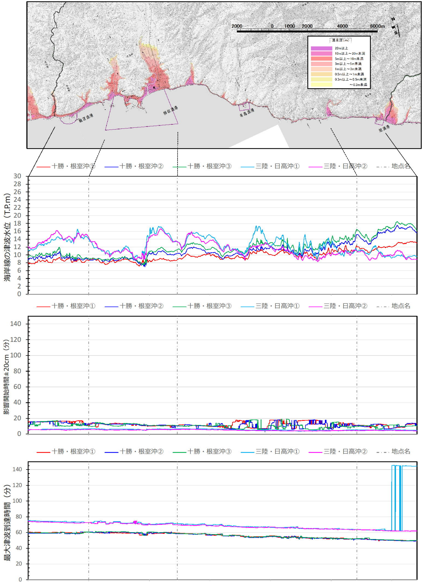
様似町 海岸線における津波水位と影響開始時間および最大津波到達時間
