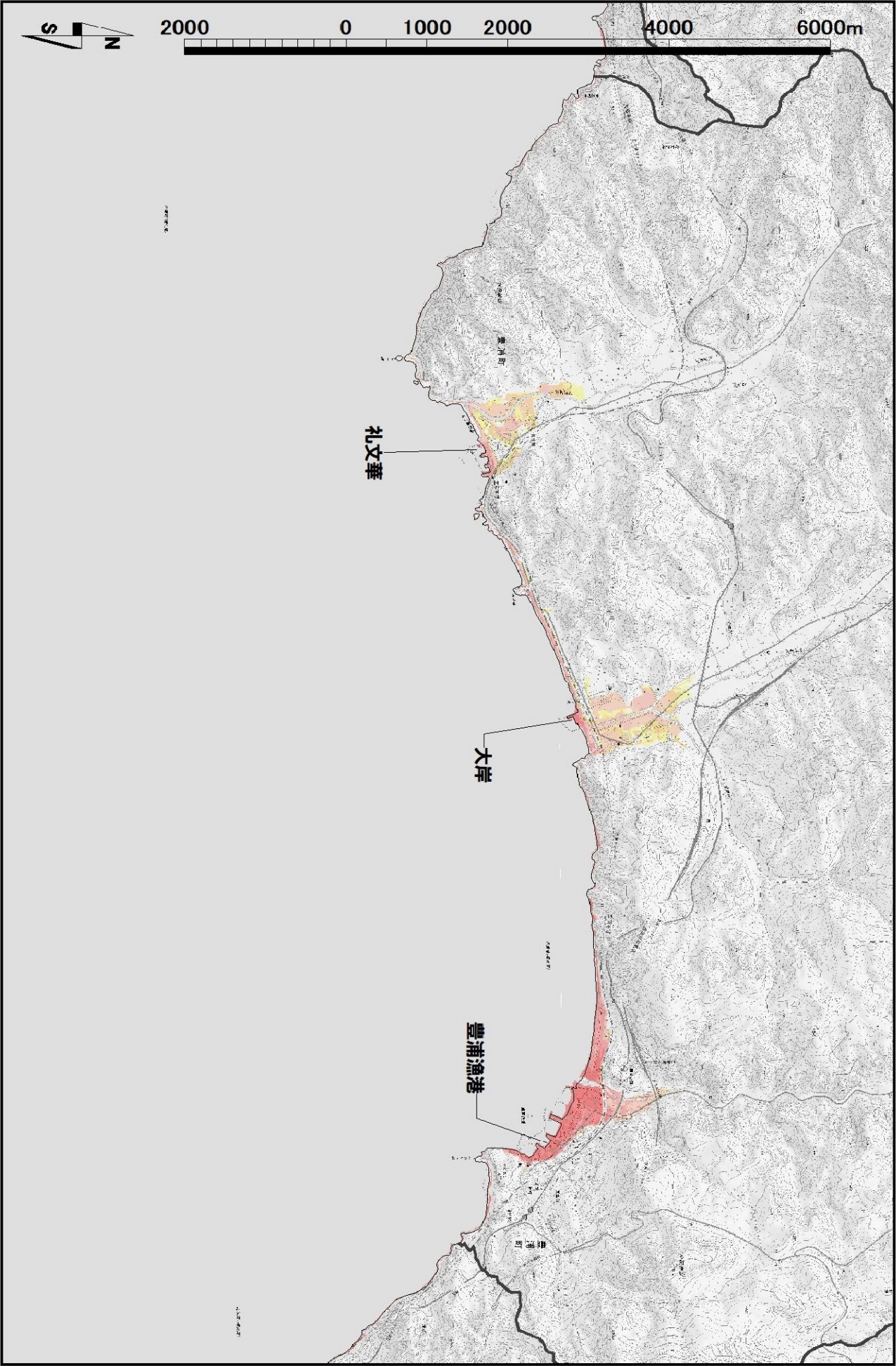
豊浦町 代表地点の津波水位時系列変化分布
