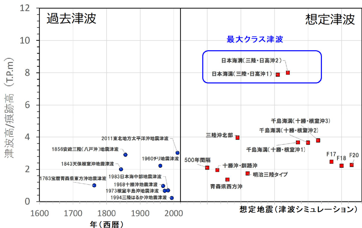
図ー5 最大クラスの津波を選定するためのグラフ(例)
