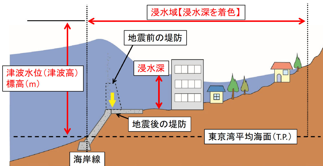
図－2 各種高さの模式図
