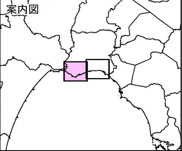
想定津波波源域
